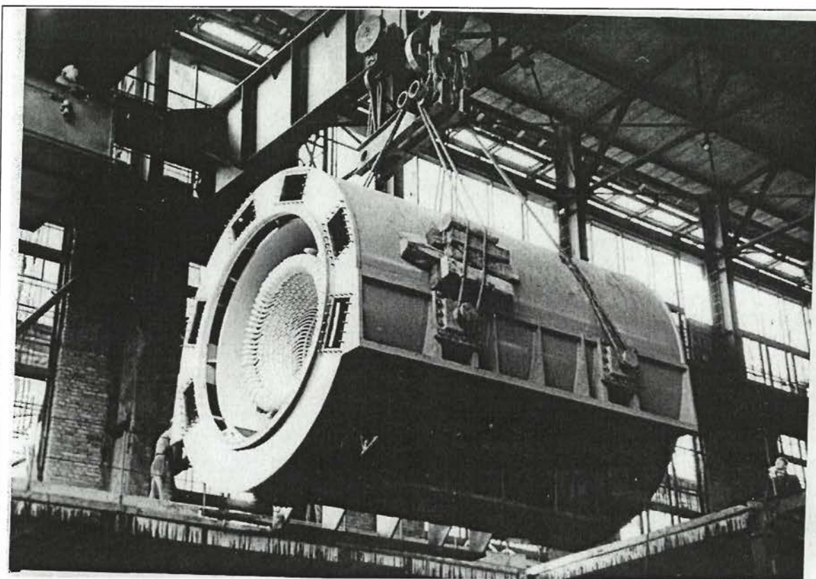
Статор над полом машзала – восьмая отметка.
