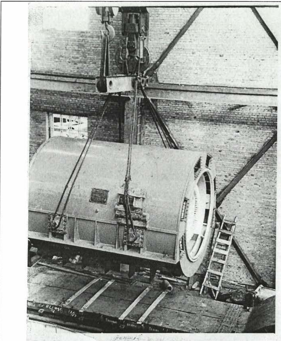
Моя траверса в работе. Подъём статора генератора мощностью 50 тыс. кВт, весом 92 тонны мостовым краном грузоподъёмностью 75/15 тонн на ТЭЦ № 20 Мосэнерго в сентябре 1958 года. Статор оторвался от спецплатформы.
